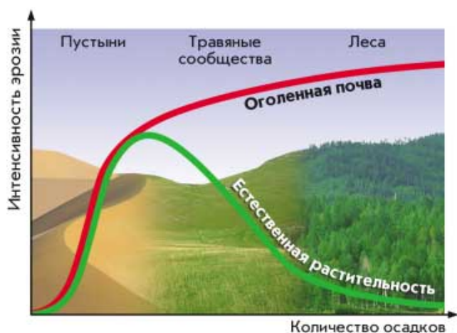
Рис. 1.15. Интенсивность эрозии почв в разных биомех (природных зонах), а также при наличии и отсутствии растительности
