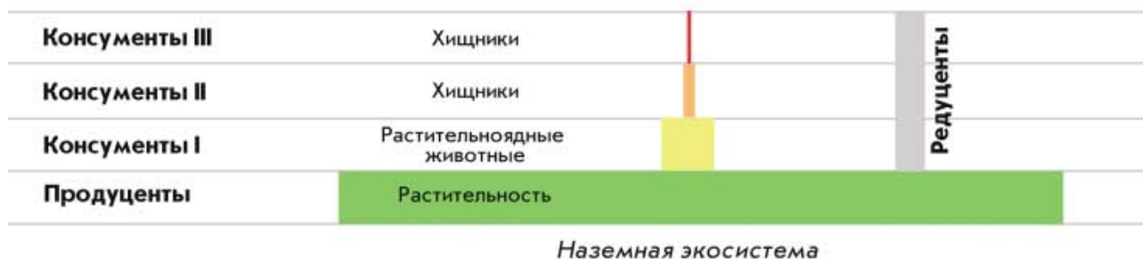
Рис. 1.3. Пирамида энергий (биомасс) в экосистеме
