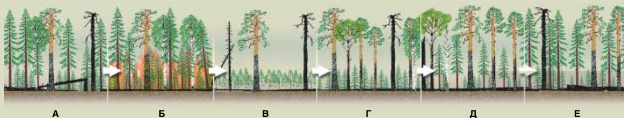
Рис. 1.26. Сосново-еловая пожарная динамика. Схема развития древостоя: А — хвойное насаждение; Б — пожар; В — послепожарный лиственно-светлохвойный подрост; Г — лиственно-светлохвойное насаждение со вторым ярусом из ели; Д — смешанное лиственно-хвойное насаждение, хвойное насаждение с распадающимся лиственным поколением; Е — хвойное насаждение
